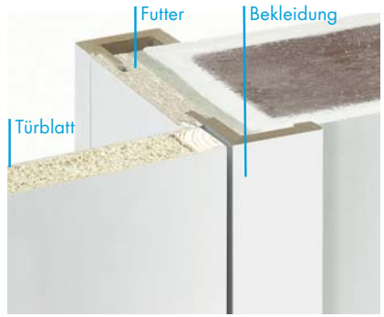
Holzfutterzarge
